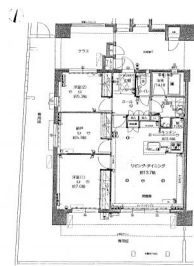
[間取り図・図面][間取り図]
